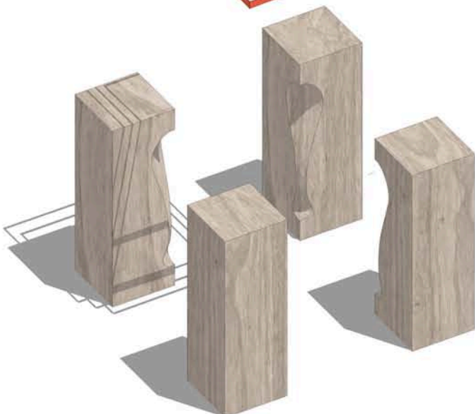
ESPLOSA ASSONOMETRICA
