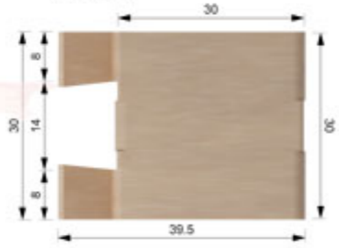
PIANTA
